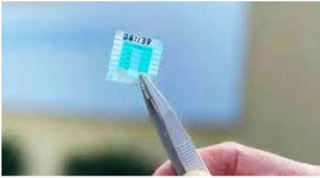
Para ilmuwan Australia telah mengembangkan prototipe baterai kuantum yang dapat menguji pengisian daya nirkabel menggunakan laser, membuka lompatan besar bagi teknologi energi.
